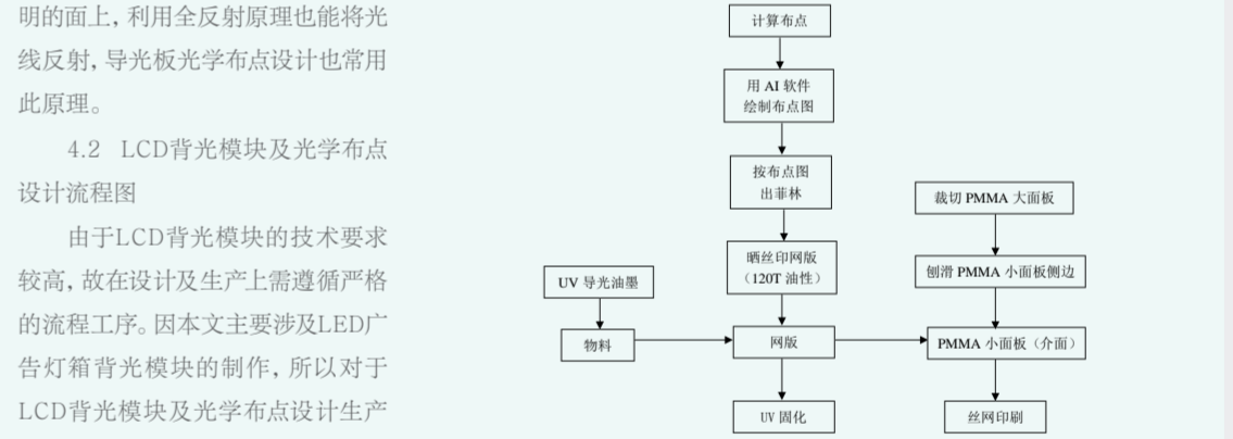
图10 制作PMMA导光板工艺流程图 (未完待续)
